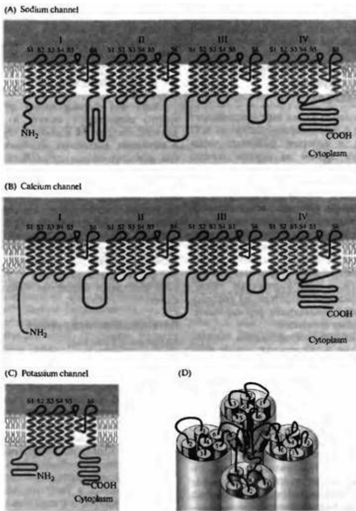
Рис. 3.6. Структура потенциал активируемых каналов. (А) Потенциал активируемые натриевые каналы, представляющие одну белковую молекулу с четырьмя доменами (I-IV), соединенными внутриклеточными петлями. Каждый домен имеет шесть трансмембранных участков (S1-S6). Структура, формирующая ионную пору, располагается между пятым и шестым сегментом. (В) Структура потенциал-активируемых кальциевых каналов подобна таковой натриевого канала. (С) Субъединица калиевого канала похожа на одиночный домен натриевого канала. (D) Предполагаемая трехмерная структура канала.
