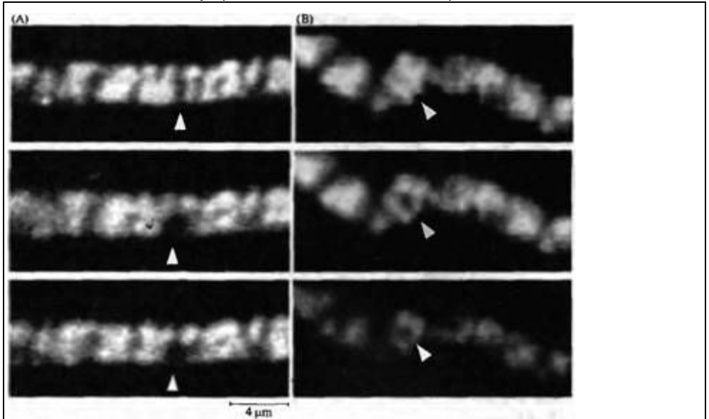
Рис. 13.17. Ограниченное движение синаптических везикул в нервной терминали. Флуоресцентные микрофотографии нервных окончаний лягушки, в которых синаптические пузырьки были помечены флуоресцентным красителем. (А) Нервное окончание до (вверху), непосредственно после (в середине) и через 28 мин после (внизу) обесцвечивания окраски в небольшом пятне в группе везикул интенсивным освещением. Обесцвеченный участок (стрелка) остается почти неизменным через 28 мин после освещения, что указывает на незначительное спонтанное перемещение окрашенных везикул. (В) То же, что и на рисунке А, за исключением того, что после обесцвечивания терминаль стимулировали током с частотой 10 Hz в течение 5 мин. Хотя группы везикул бледнели, так как высвобождали окрашенное содержимое в ходе экзоцитоза, этот процесс не затрагивал обесцвеченный участок, что говорит об отсутствии передвижения окрашенных везикул в эту область.
